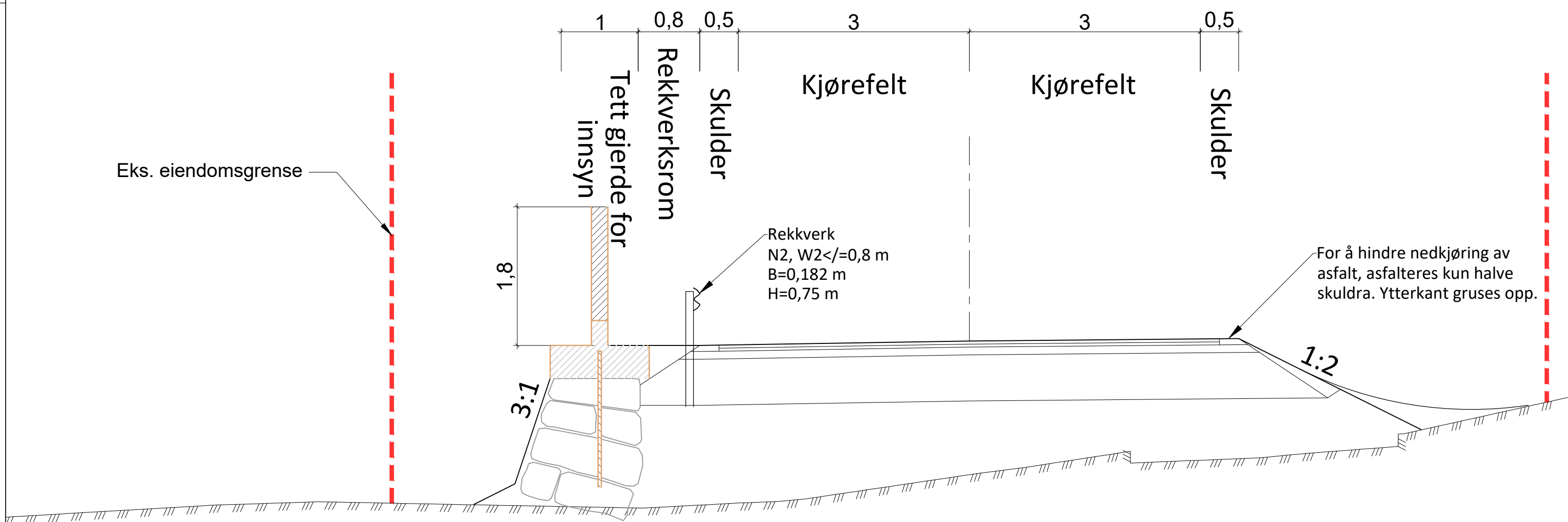
Normalprofil Profil 20 langs Storbuktveien
