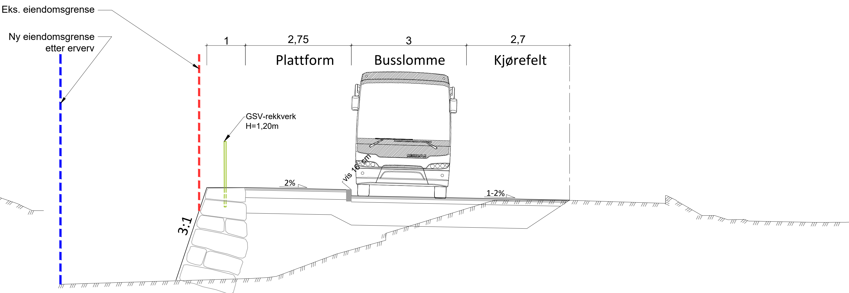
Normalprofil Profil 30 langs Kvalvikveien
