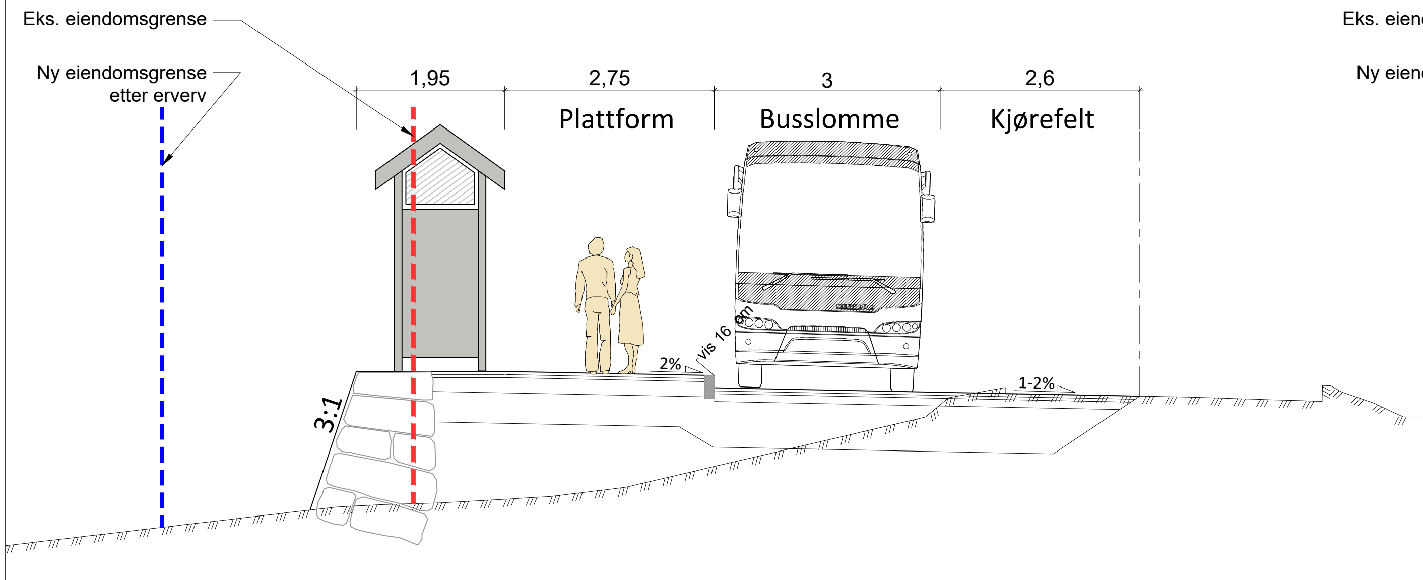
Normalprofil Profil 26 langs Kvalvikveien
