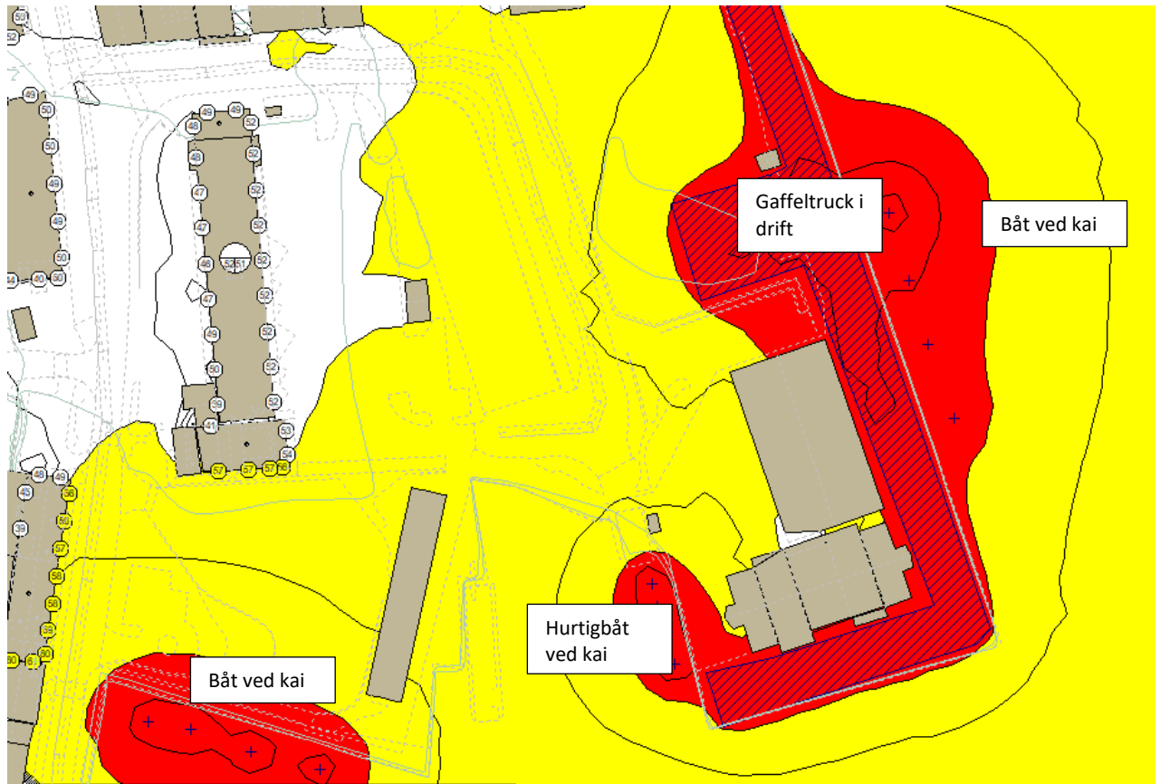
Figur 4: Støysonekart, L_{den} 4 meters høyde.
